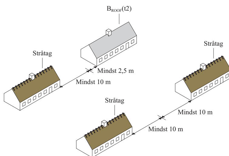
Figur 7.4. Afstanden mellem enfamiliehuse på samme grund, hvis et eller flere af bygningerne har tagdækning, som ikke er tagdækning klasse B_{ROOF}(t2) [klasse T tagdækning].
