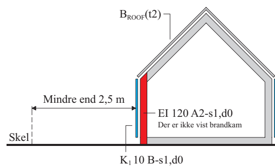
Figur 5.11. Afstande til skel.
