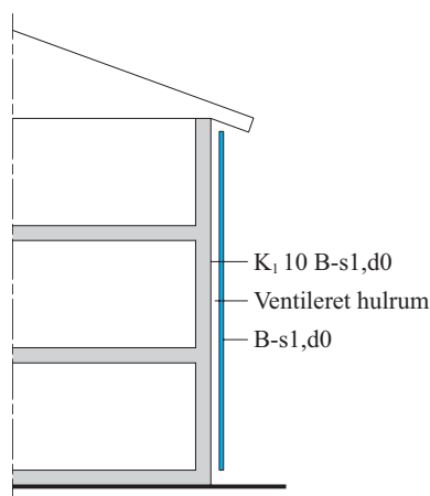
Figur 5.3. Regnskærm.
