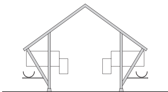
Figur 8.4. Staldopbygning.
