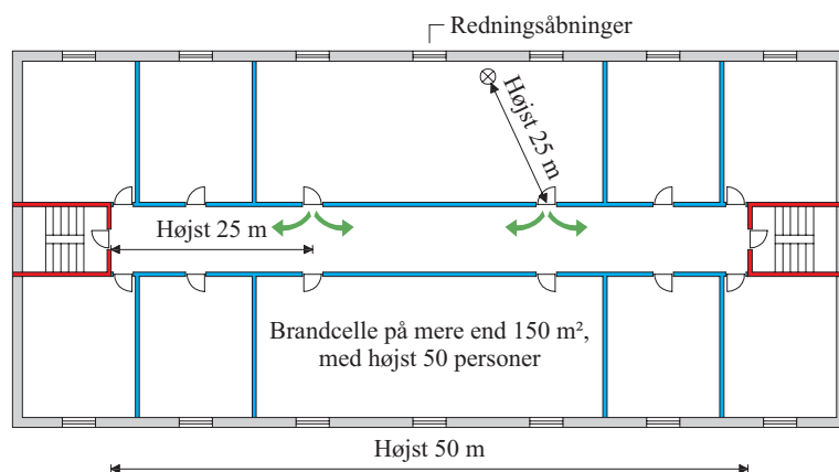
Figur 2.1. Døre til flugtveje fra brandcelle over 150 m² og med højst 50 personer.
