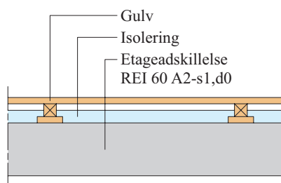
Figur 3.1. Etageadskillelse.
