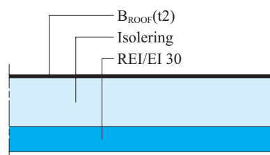
Figur 3.3. Tagkonstruktion.
